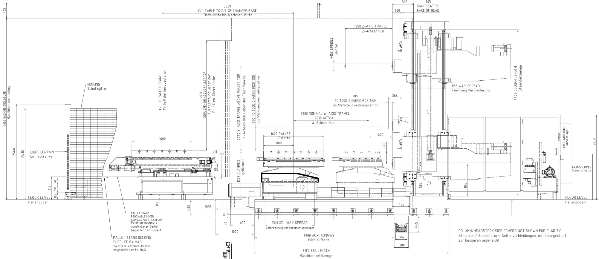
RIGHT SIDE VIEW Ansicht rechte Seite
